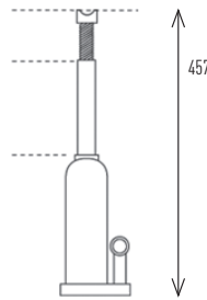
TL108N / 8 TON
