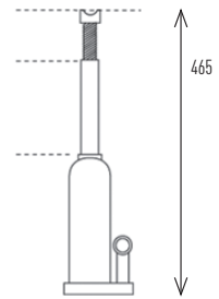
TL112N / 12 TON
